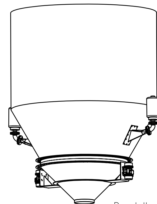
Darstellung ohne Einhausung Maßstab 1:50
