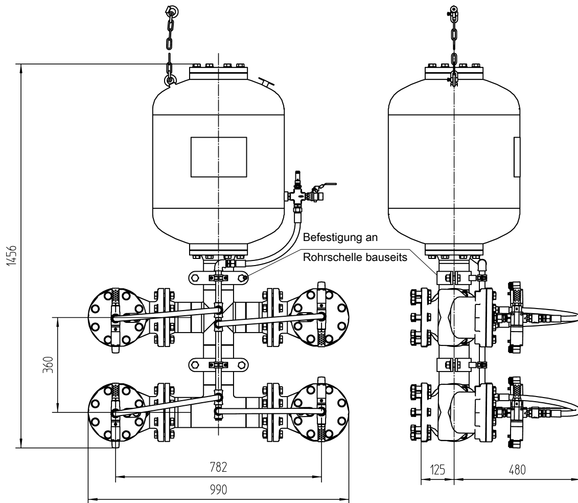
Abb. 1: Maßblatt PP-4 AVE-2 Typ BB
