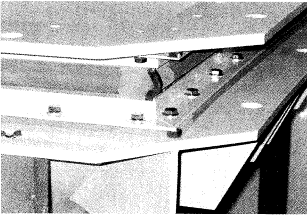
Bild 2: Die besondere Abdichtung des VIBOSTAR® Schwingtrichters.
