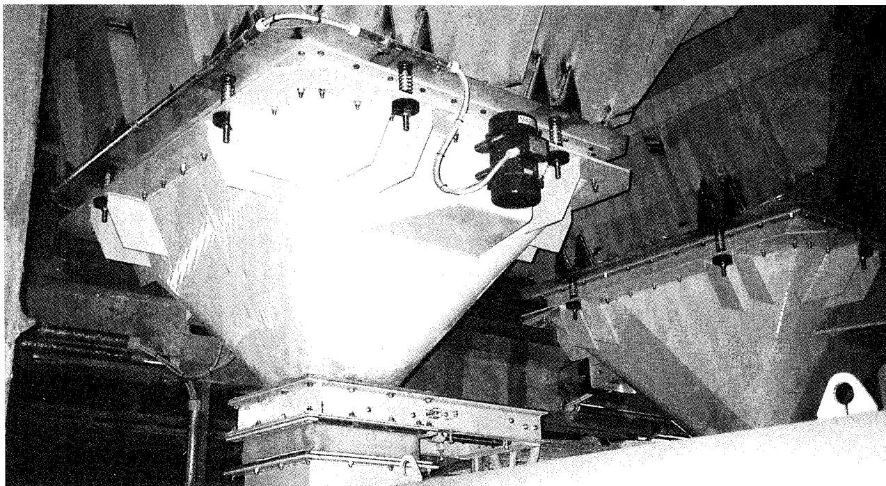
Bild 1: Rechteckige VIBOSTAR® Schwingtrichter zum Austrag von Hüttensand und Zement.
